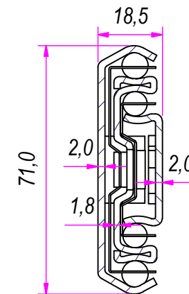
SEZ. A-A
