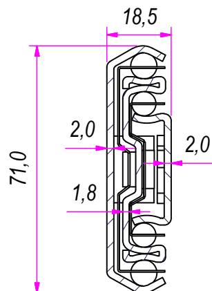
SEZ. A-A
