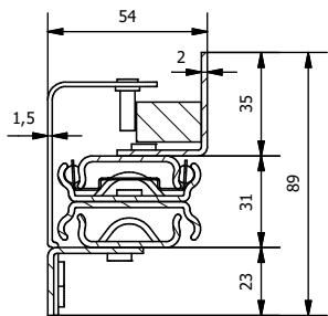
A-A (1:2)
