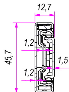
SEZ. A-A
