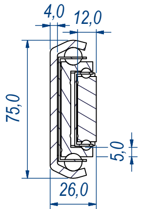
SEZ. A-A
