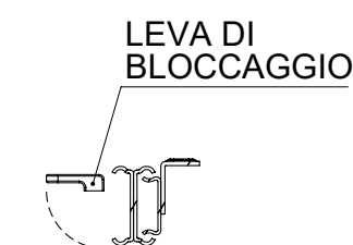
SEZIONE C-C
