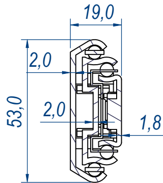
SEZ. A-A
