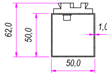
SEZ. A-A
