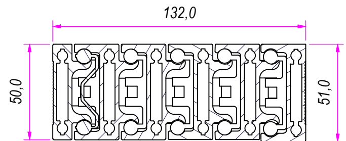
SEZ. A-A
