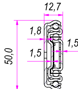
SEZ. A-A
