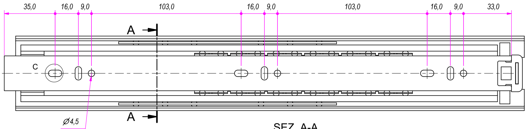
SEZ. A-A
