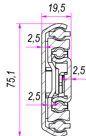
SEZ. A-A
