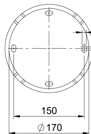
DETTAGLIO B SCALA 1:5
