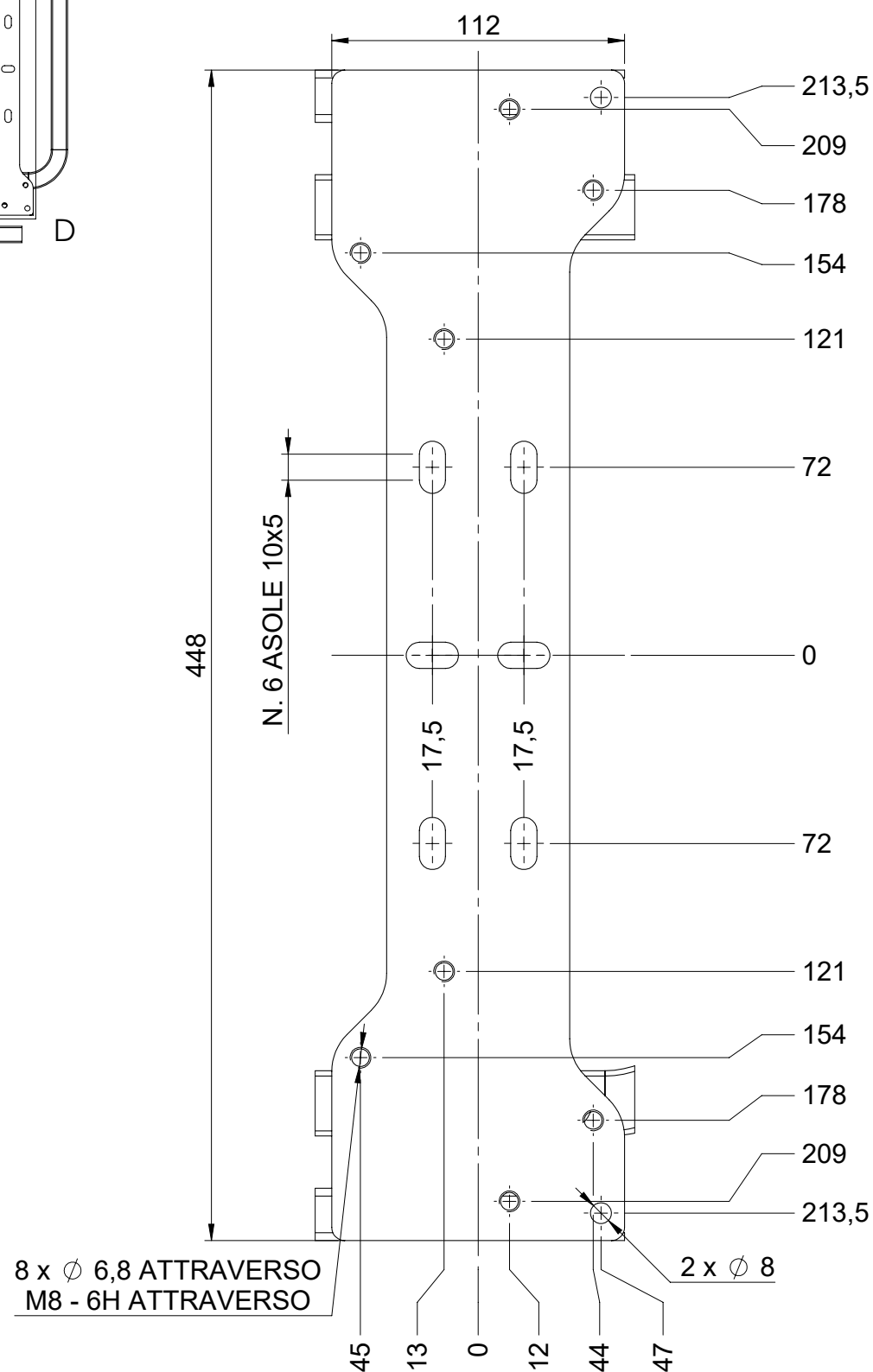
DETTAGLIO D SCALA 1:2,5
