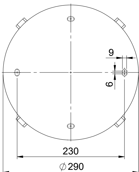
DETTAGLIO A SCALA 1:5
