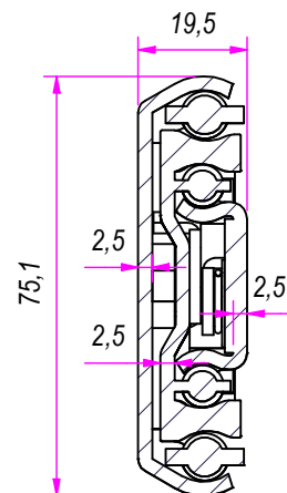
SEZ. A-A
