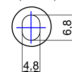
E (1:1)
